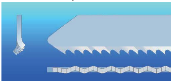
frézované vlnité zuby
