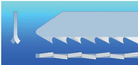
frézované bočné zuby
